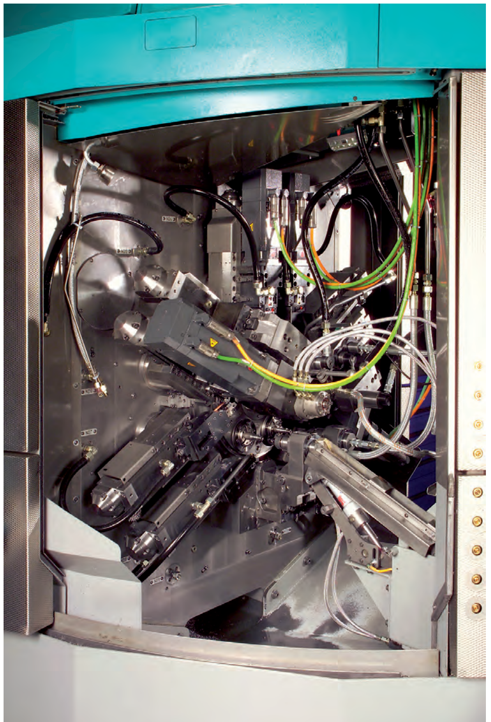
Drehautomat bei Firma Wagner
